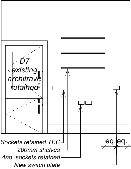
Elevation B
