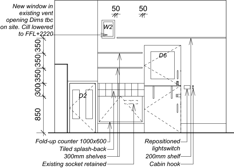
Elevation A
